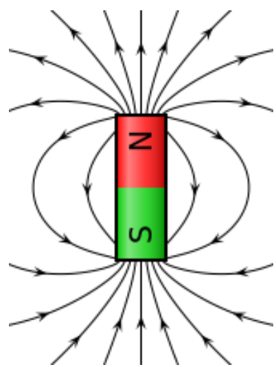
Мал.: Внутрішній стрижневий магніт Землі (Джерело: Geek3, https://de.wikipedia.org/wiki/Magnetismus )
