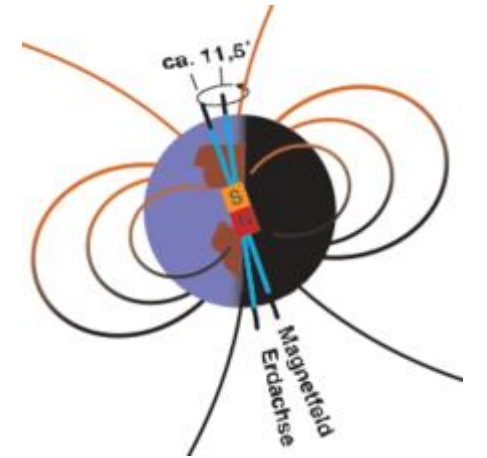
Мал.: Магнітне поле Землі (Джерело: GFDLХубі, https://de.wikipedia.org/wiki/Pol_(geomagnetismus) )
